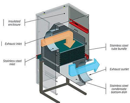
Τοποθέτηση Εναλλάκτη
