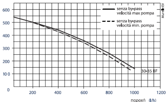
Διαθέσιμο Μανομετρικό (mbar)
