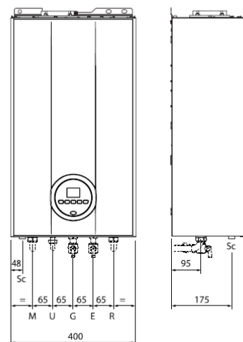
Διαστάσεις - Υδραυλικές συνδέσεις
