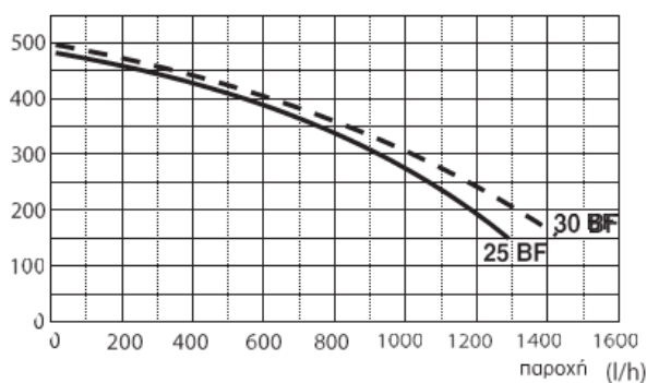
Διαθέσιμο Μανομετρικό (mbar)
