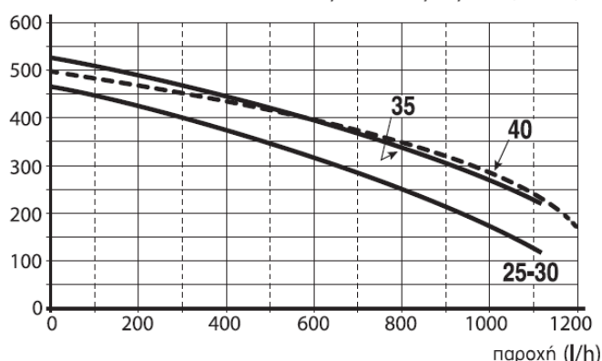
Διαθέσιμο Μανομετρικό (mbar)
